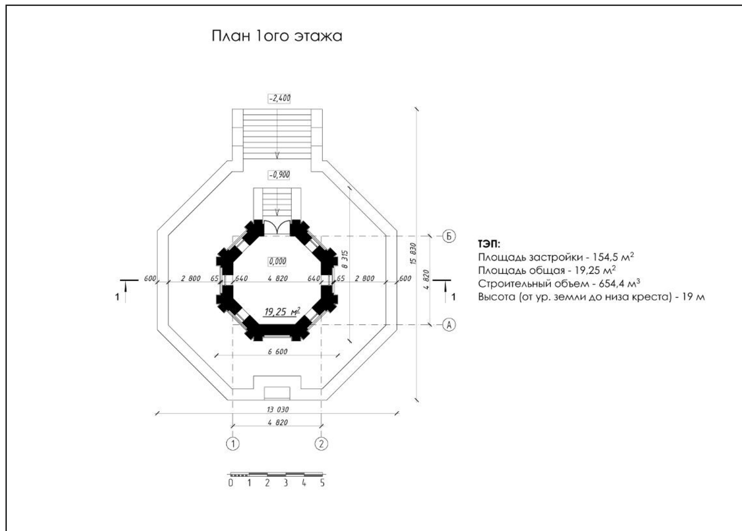
Илл. 28. Нижегородская область, г. Нижний Новгород, воссоздание Алексеевской часовни при Благовещенском монастыре - 2026 г. План 1-го этажа (предоставлен заказчиком).
