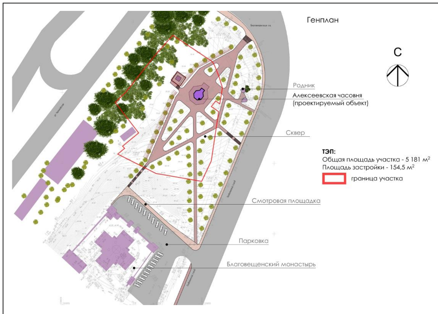
Илл. 27. Нижегородская область, г. Нижний Новгород, воссоздание Алексеевской часовни при Благовещенском монастыре - 2026 г. Схема генерального плана (предоставлена заказчиком).
