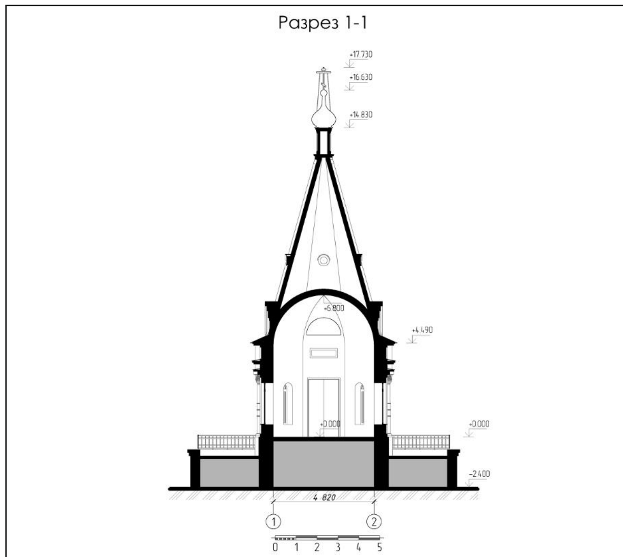
Илл. 29. Нижегородская область, г. Нижний Новгород, воссоздание Алексеевской часовни при Благовещенском монастыре - 2026 г. Разрез 1-1 (предоставлен заказчиком).
